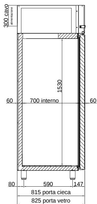
SEZIONE A-A
