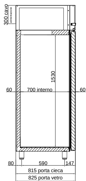
SEZIONE A-A
